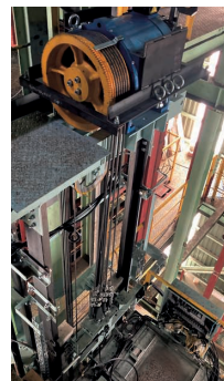
省スペースの巻上装置
